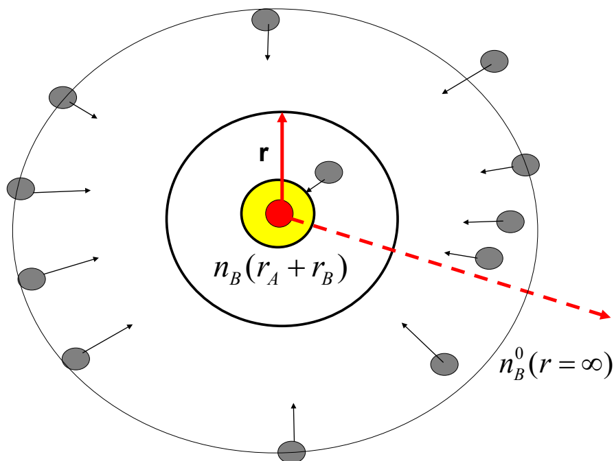
Рис.1. Модель Смолуховского. Красный кружок – частица А, серые кружки– частицы В. Желтым обозначена реакционная зона, где концентрация В равна n_{B,(r_A+r_B)} . Концентрация В растет по мере удаления от А одинаково во всех направлениях (например, вдоль красной пунктирной линии) и достигает значения n_B^0(r = \infty) , средней концентрации В в растворе.
