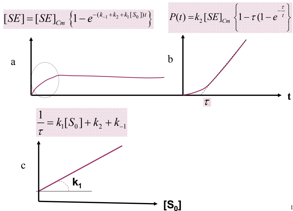
Рис.1. Расчет параметров уравнения Михаэлиса – Ментен.
